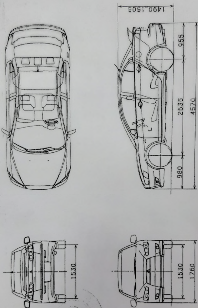
Общий вид автомобиля MITSUBISHI Lancer (CY0)
